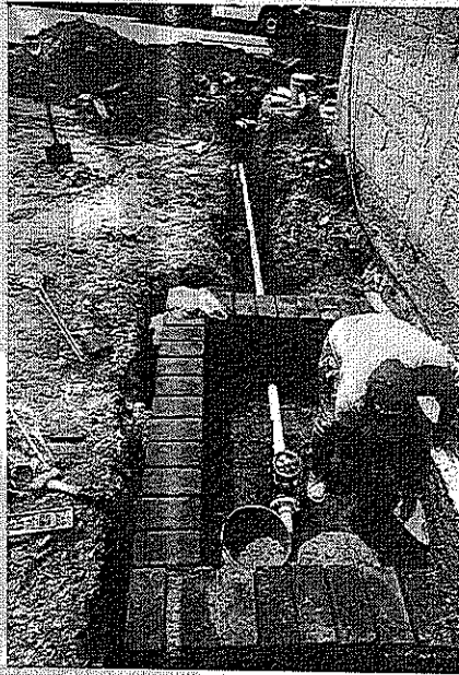
Construcción de red de agua potable en calle Lago Zumpango, colonia El Cueyamil
